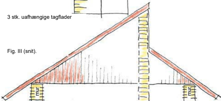
2 stk. uafhængige tagflader
